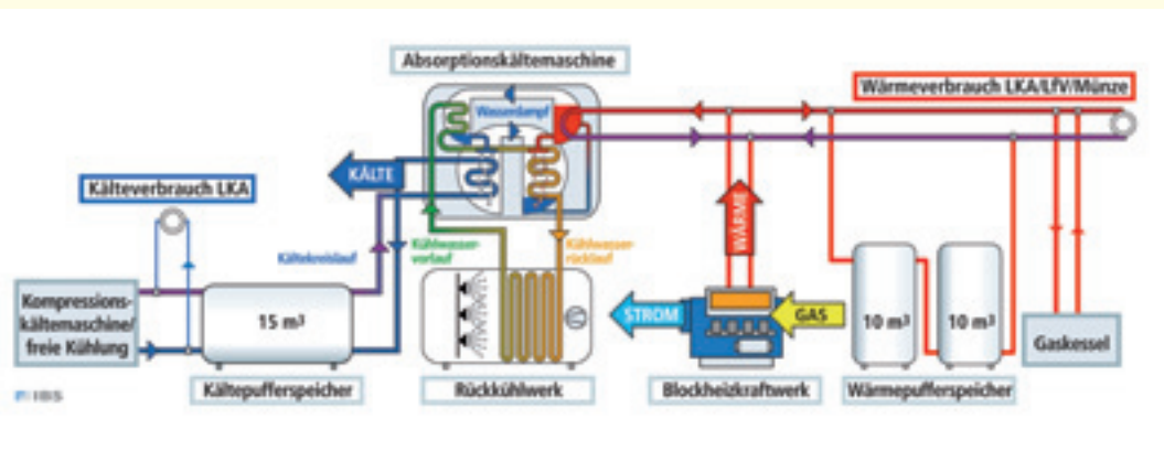
Anlagenschema Kraft-Wärme-Kälte-Kopplung Blockheizkraftwerk mit Absorptionskältemaschine im Landeskriminalamt Baden-Württemberg
